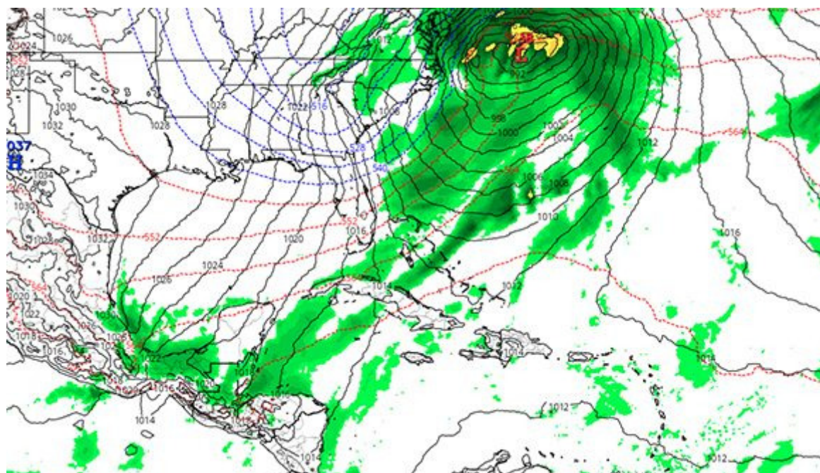
Frente frío transitando por el territorio cubano durante el sábado 29 de enero, según modelo ICON. Imagen: tomada de MeteoAlerta.
